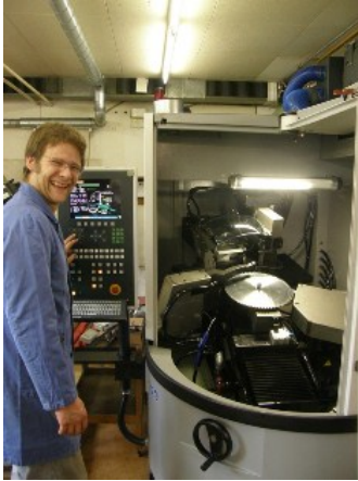
Vollmer CL200 Unsere neueste Anschaffung. CNC-gesteuerte 5-Achsen-Maschine Zum Schärfen von HM-Kreissägen in einer Aufspannung.
