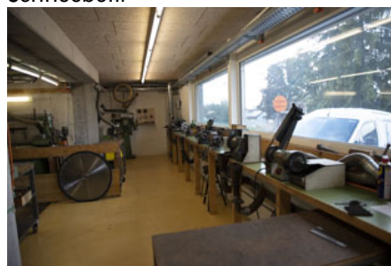
Vollmer CV-Sägen-Schärfmaschine, automatisiert durch Max Schneebeli.
